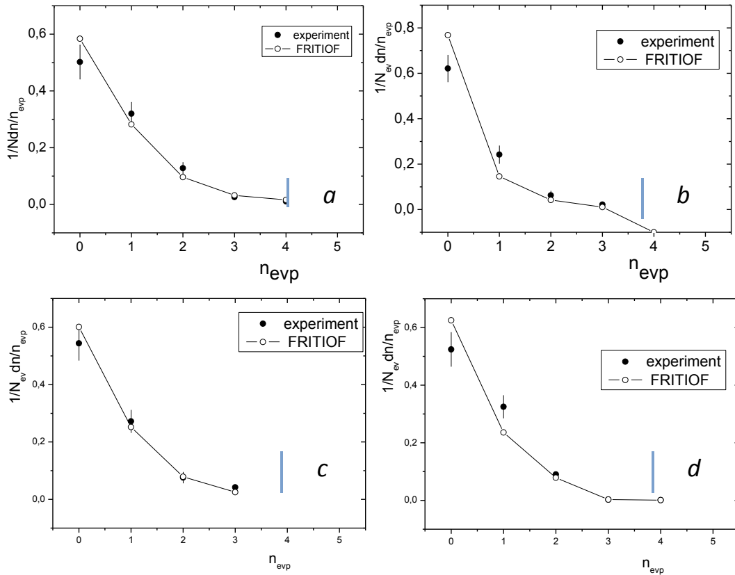
Рис.3. Множественное распределения испарительных протонов в СС-взаимодействиях. а) n_p^{yч} \leq 4 , б) 4 \leq n_p^{yч} \leq 9 , в) n_p^{yч} > 9 , д) Q_{стр}=0 .
